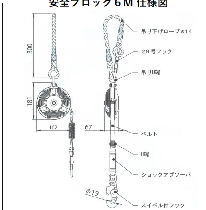
安全ブロック 6 M 仕様図
